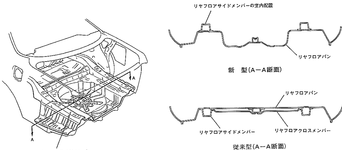
リアフロアサイドメンバーの室内配置
