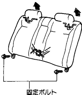
固定ボルト
