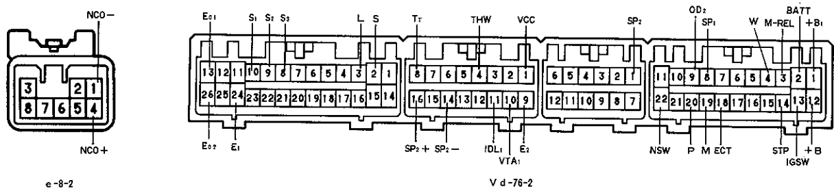
エンジンコントロールコンピューター(7 M-GE)
