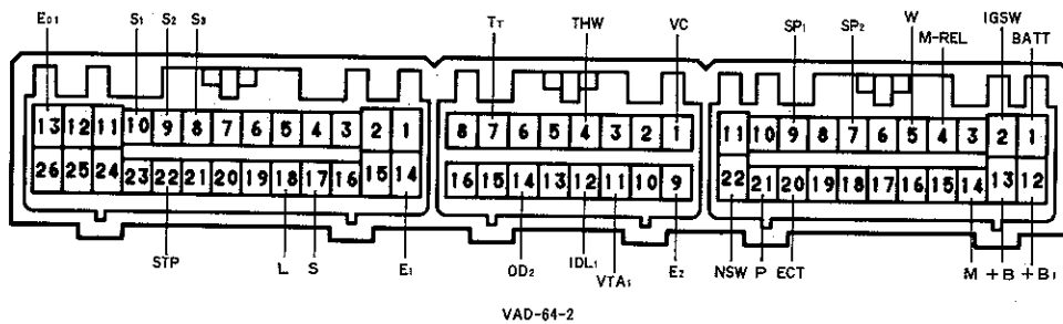
エンジンコントロールコンピューター(7 M-GE)
