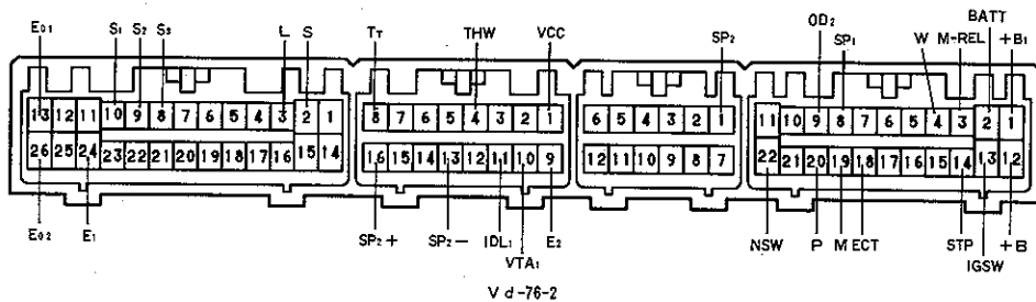
エンジンコントロールコンピューター(1 JZ-GTE)
