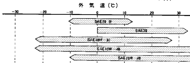
SAE粘度分類と使用可能な外気温度との関係
