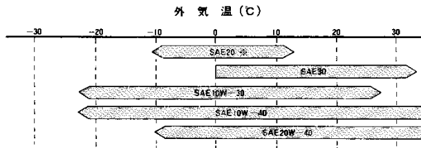
SAE粘度分類と使用可能な外気温度との関係
