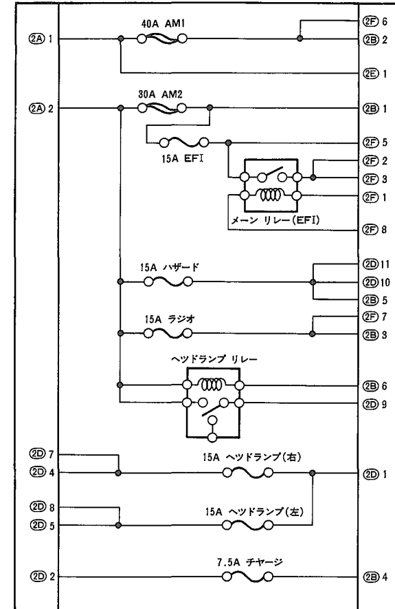
J/B No.2内部回路図
