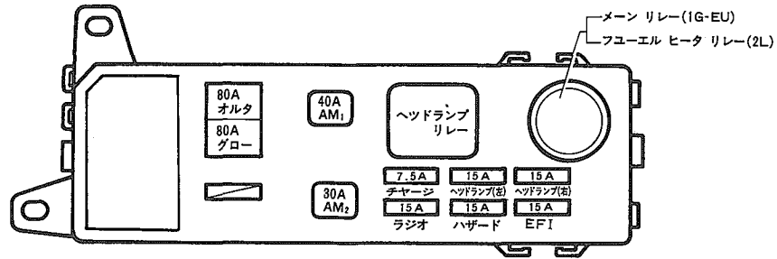
J/B No.2(エンジン ルーム)
