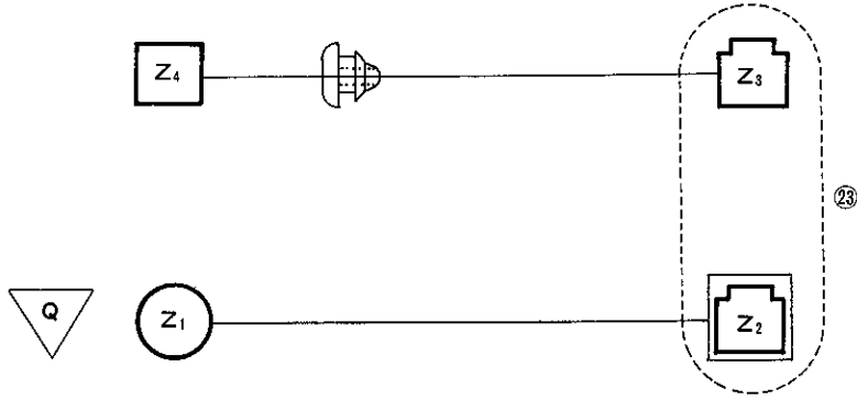
図24-1 ワイヤ, リヤ ウインド デフォガ
