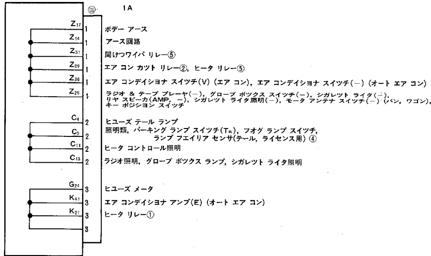
リレー ブロック内回路図
