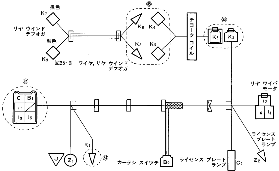
③④ ..... 図23 ワイヤ, ランプ(リヤ用)へ
