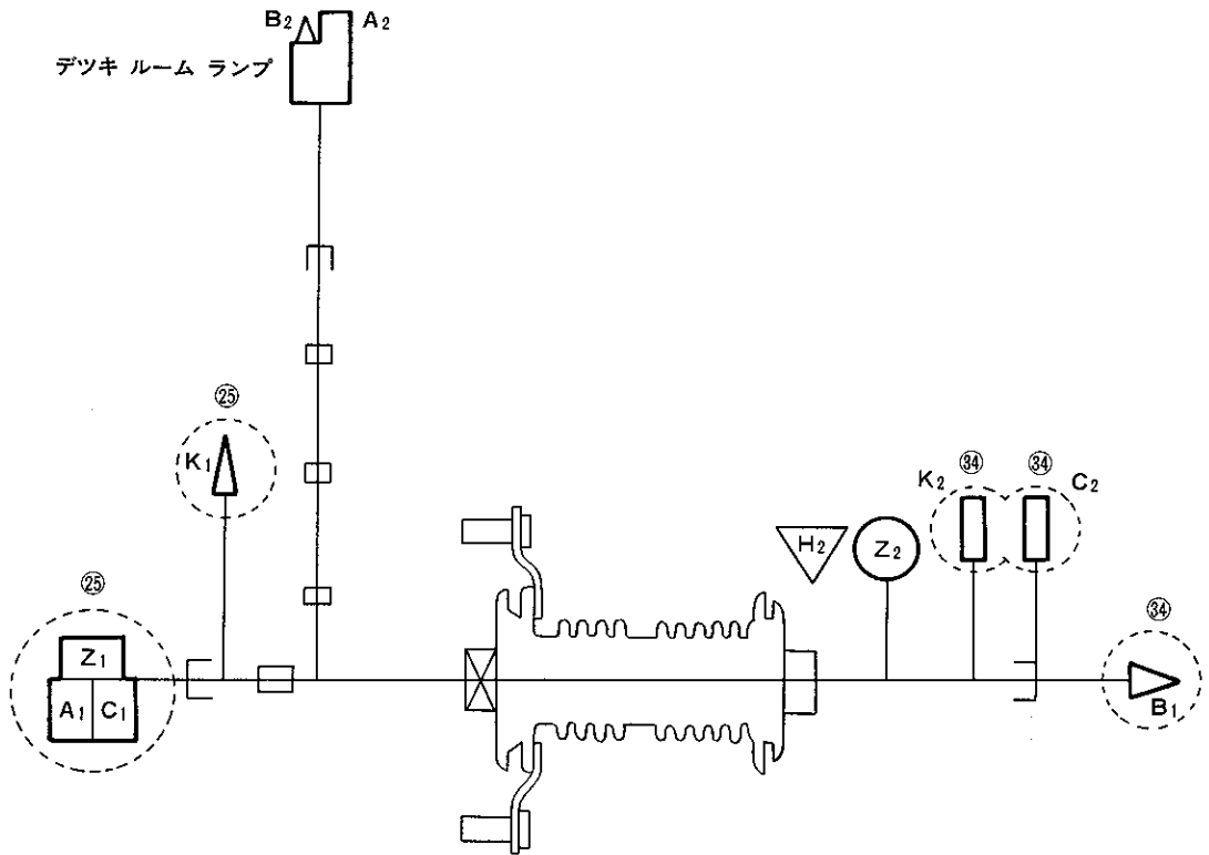
図23-1-1 ワイヤ, ランプ(リヤ用) (バン<STD, DX>)
