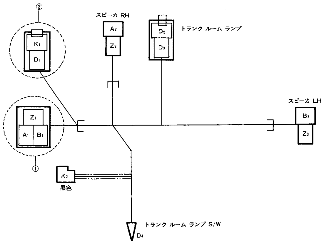
図6-2 ワイヤ, ツウ ラジオ インストレーション (コロナ マークII セダン-L[ステレオ付き], LG, LGツーリング チエイサー セダン-SXL[ステレオ付き], SGS[ステレオ付き], SG ツーリング)
