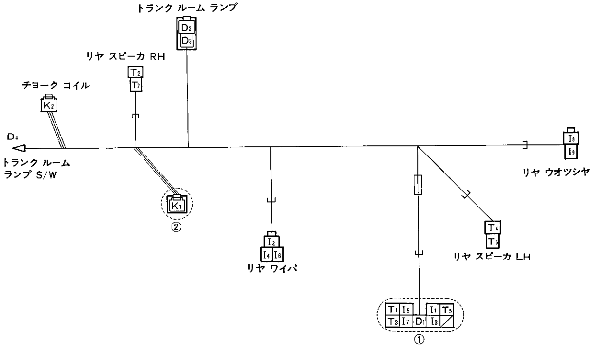
図7-1 ハーネス ASSY, ワイヤリング ツウ リヤ ランプ (コロナ マークII セダン—グランデ)
