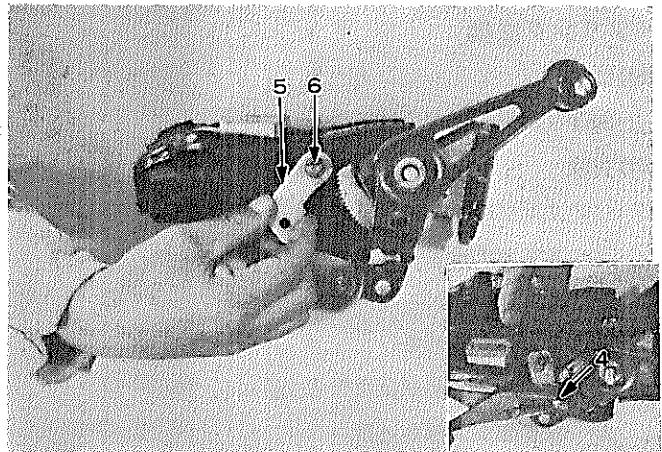
図12-47 テルトステアリングポール取りはずし
