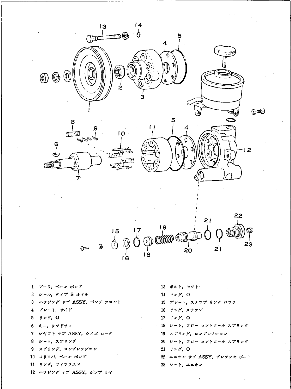
図12-93 構成部品および締め付けトルク
