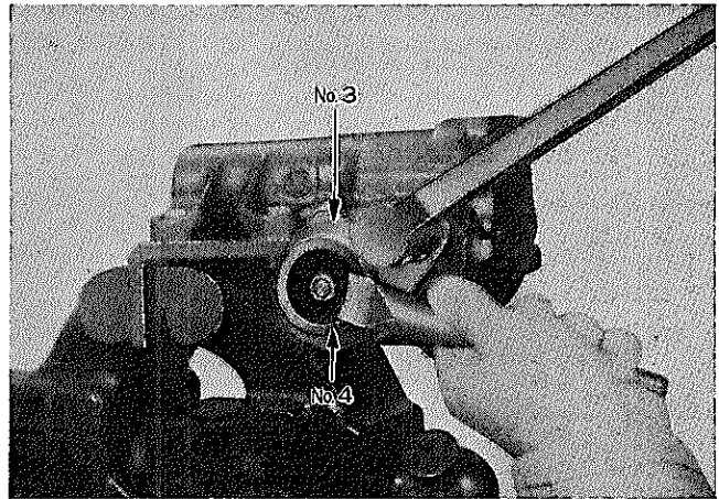
図12-147 ロック ナット締め付け
