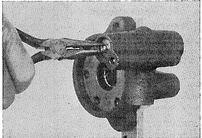
図12-100 スプリングシート取りはずし
