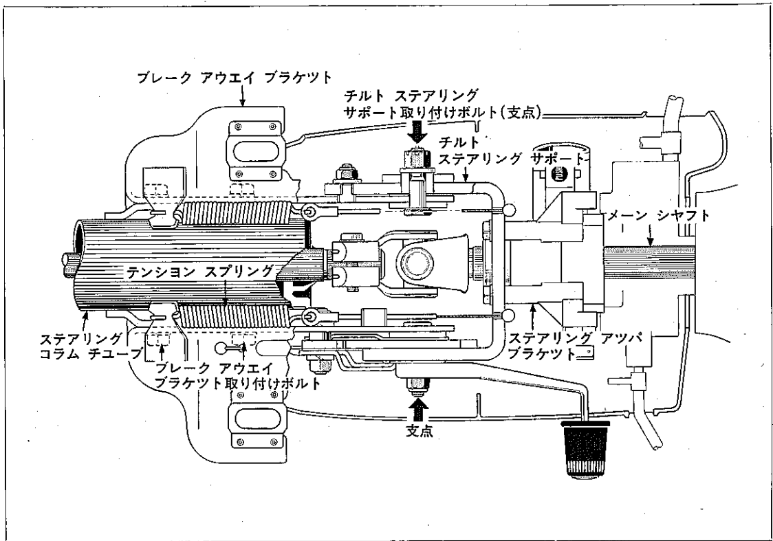
図12-30 チルト ステアリングの構造
