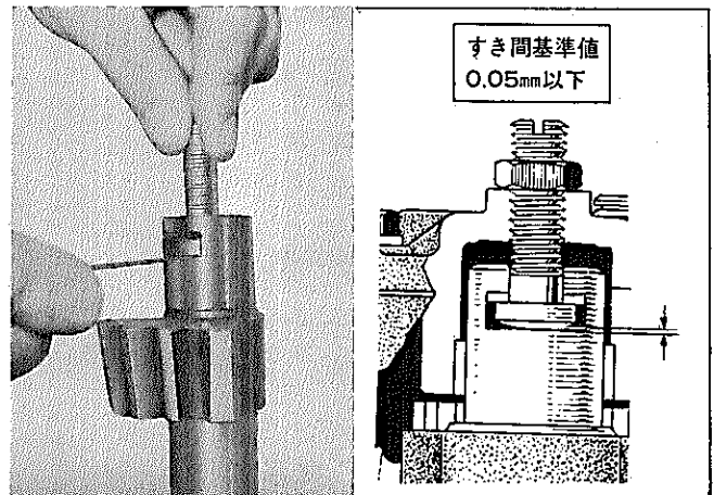
図12-67 スラストすき間測定
