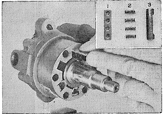
図12-120 スリツバ組み付け
