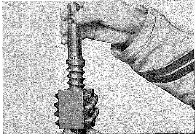
図12-66 ウォーム点検 (その2)
