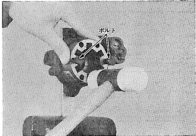
図12-118 フィックスドリング組み付け
