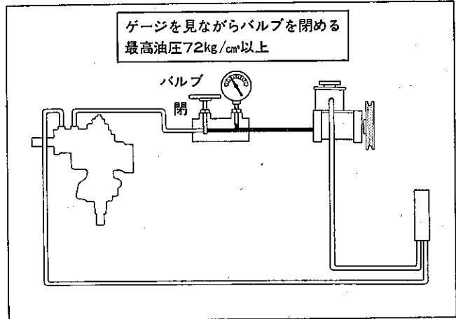
図12-90 油圧測定
