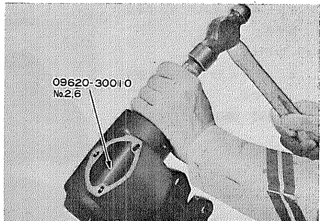
図12-73 ベアリング カップ取り付け
