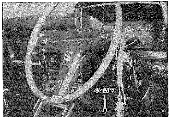
図12-92 据切り操だ力点検
