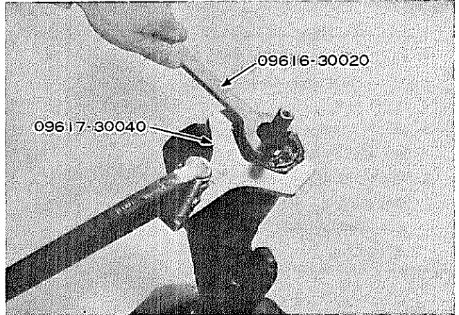
図12-77 ロック ナット締め付け
