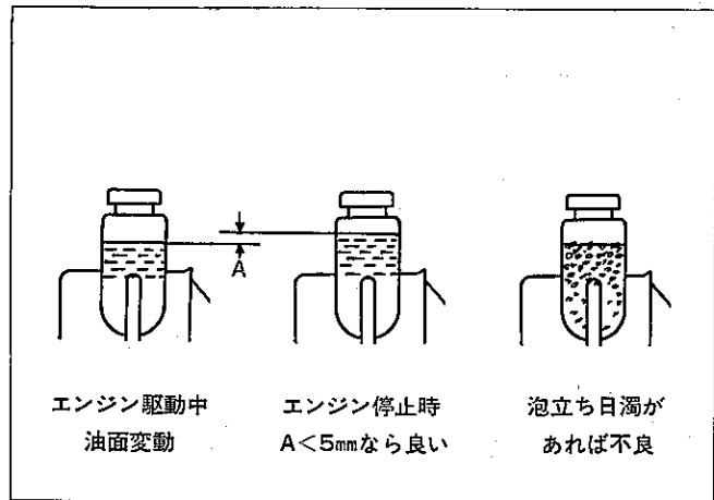
図12-87 フルード判定
