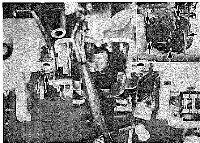
図12-34 取りはずし (運転席側)
