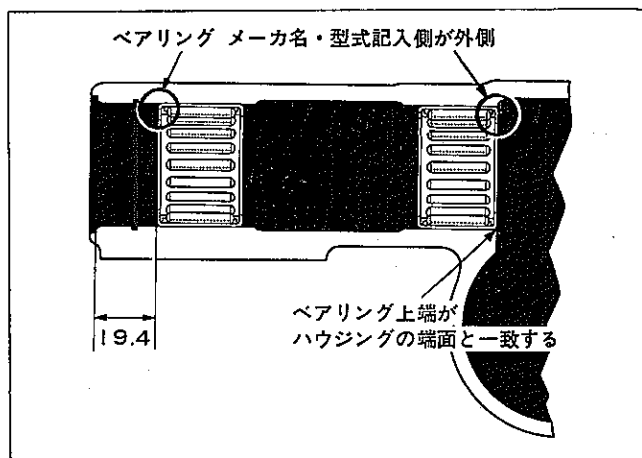
図12-143 ベアリング取り付け位置
