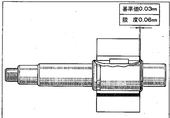
図12-104 フィットクスド リング長さ<ロータ長さ
