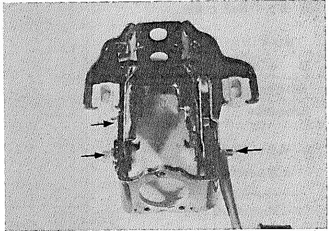
図12-48 セレクション ボルト取りはずし
