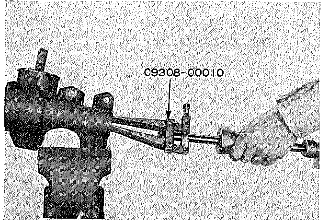
図12-68 オイル シール取りはずし
