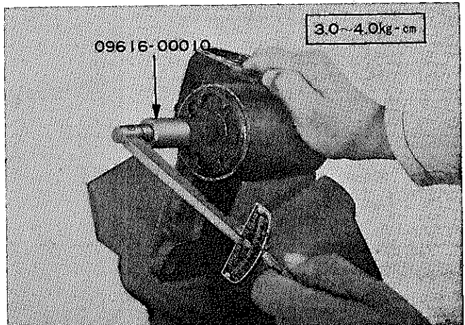
図12-76 起動トルク測定
