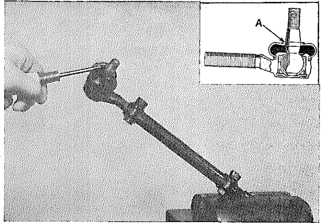
図12-168 ダスト シール交換
