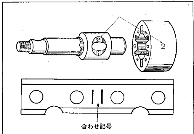
図12-119 合わせ記号
