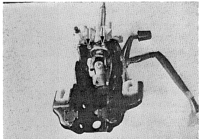
図12-38 ステアリング コラム アツパ ブラケットと チルト ステアリング サポート切り離し
