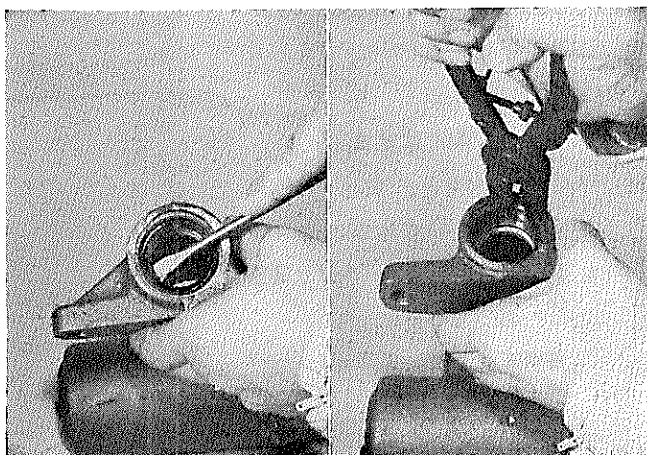
図12-136 スナツプ リング取りはずし
