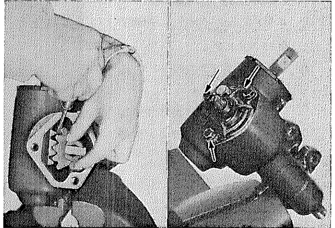
図12-78 セクタ シャフト & エンド カバー組み付け
