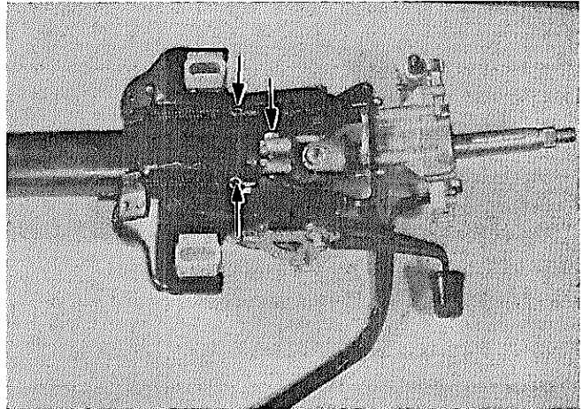
図12-36 インタミューデイト シャフトと メー ン シャフト切り離し
