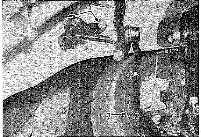
図12-171 組み付け
