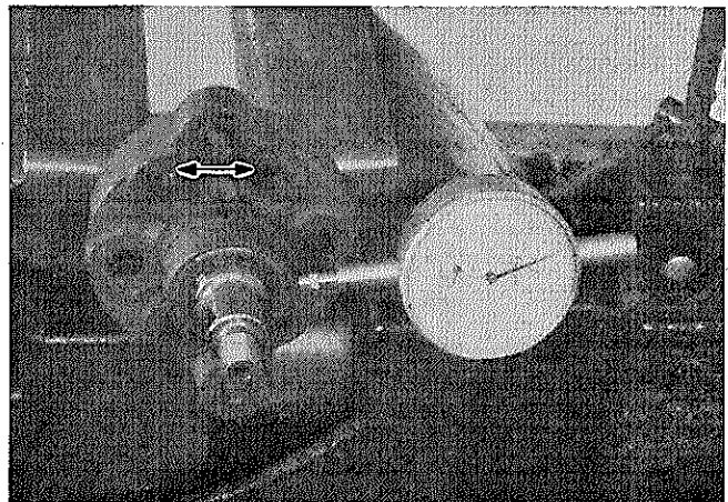
図12-107 ハウジング ブシユ摩耗点検 C0250
