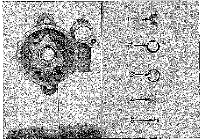
図12-114 スプリングシート組み付け
