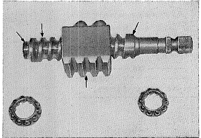
図12-65 ウォーム点検 (その1)
