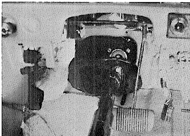
図12-35 ステアリング コラム抜き出し
