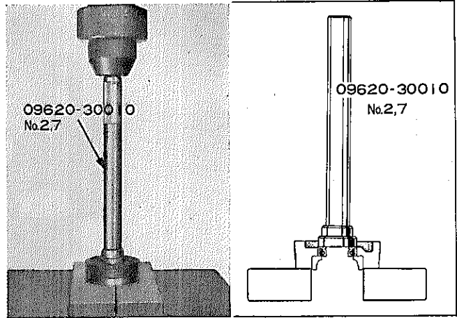
図12-71 ベアリング カップ取りはずし
