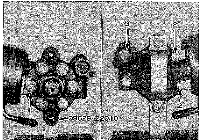
図12-97 オイル リザーバ取りはずし
