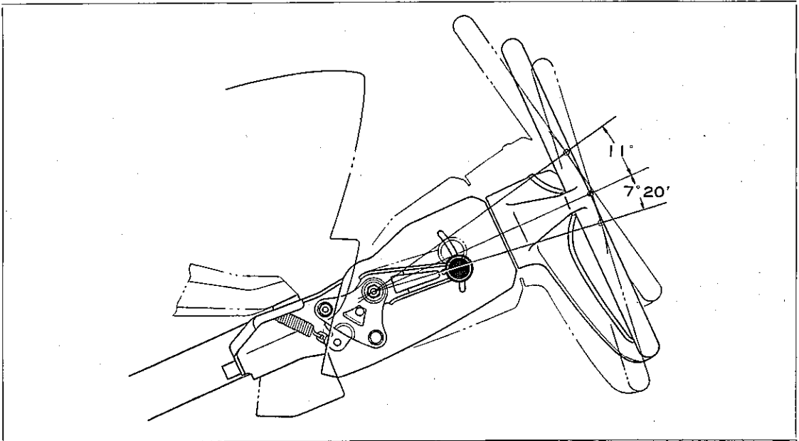
図12-29 チルト ステアリング装置
