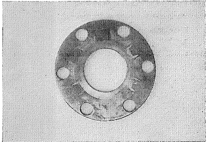
図12-106 サイドプレート点検 C0249
