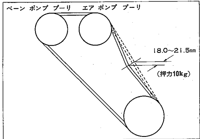
図12-86 V ベルト張り点検
