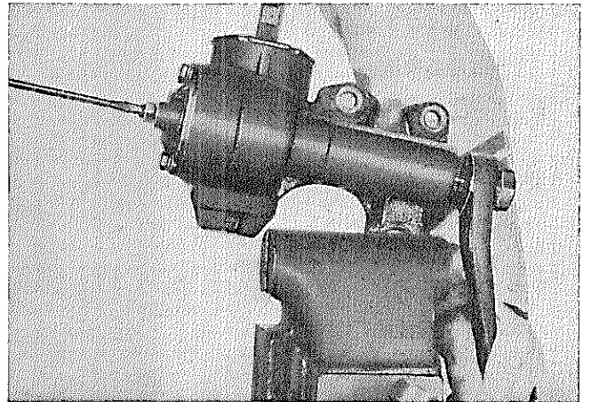
図12-79 アジャステイニング スクリユ締め込み
