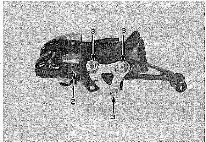
図12-46 テルトレバーリテーナ取りはずし
