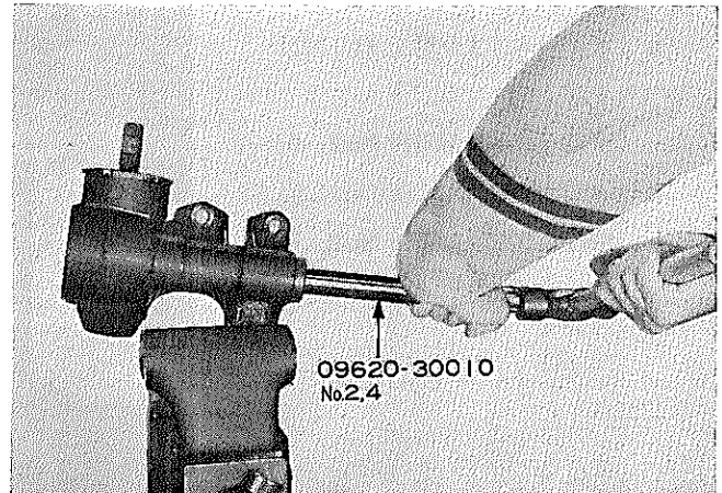
図12-69 オイル シール取り付け
