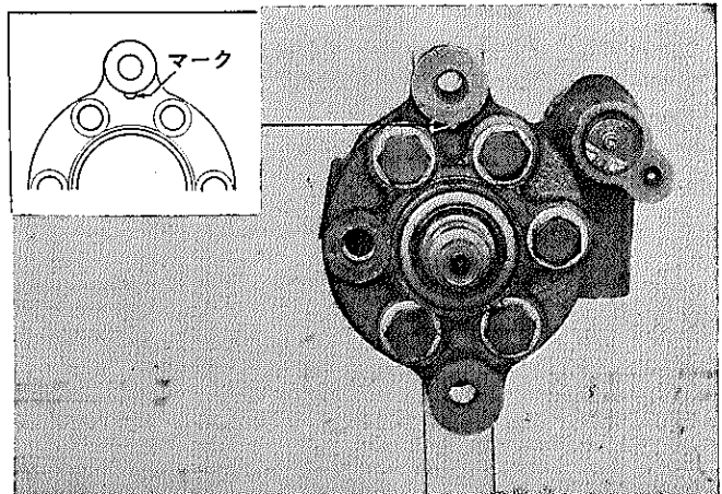
図12-122 フロントハウジング組み付け
