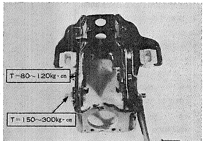
図12-53 チルト ステアリング サポート組み付け
