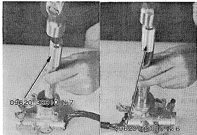
図12-44 アツパ ベアリング交換 H1323 H1324
