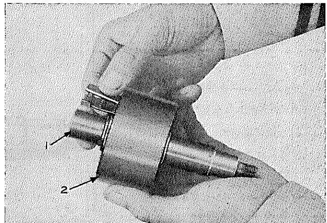
図12-101 スリツパ取りはずし
