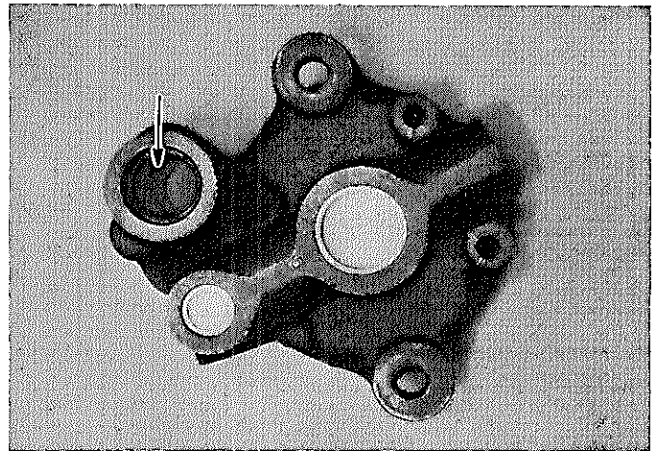
図12-109 コントロールバルブそう入部点検
