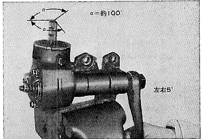
図12-81 バックラッシュ確認
