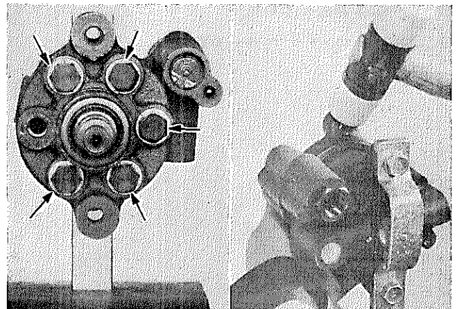
図12-98 フロントハウジング取りはずし
