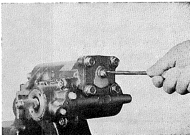
図12-153 アジャステイニング スクリュ締め込み
