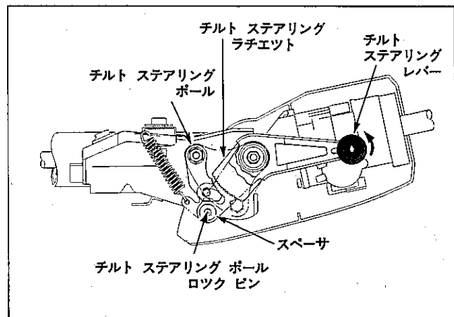
図12-32 チルト ステアリングの作動 (その2) M3458
