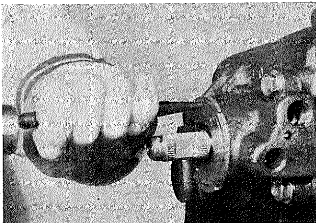
図12-155 カシメ
