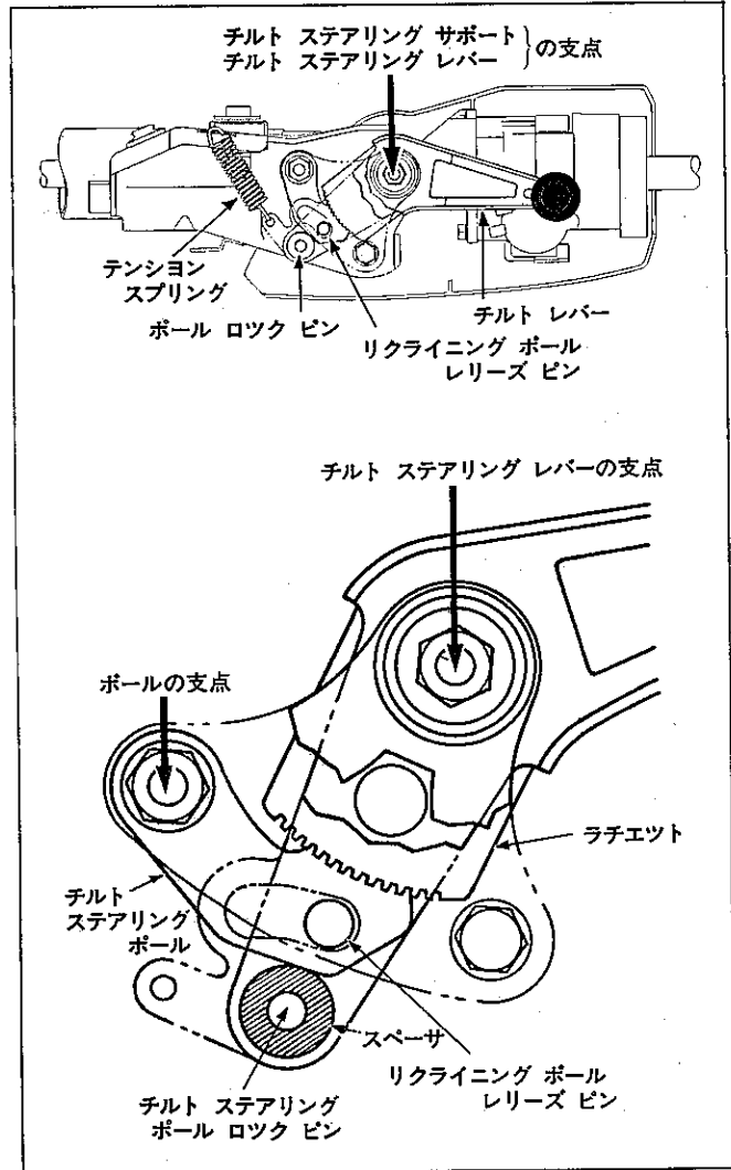
図12-31 チルト ステアリングの作動 (その1) M3456 M3457
