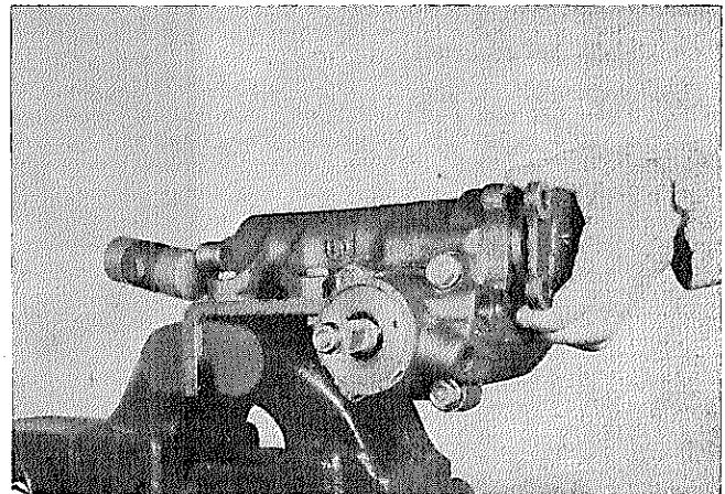
図12-131 クロスシャフト取りはずし
