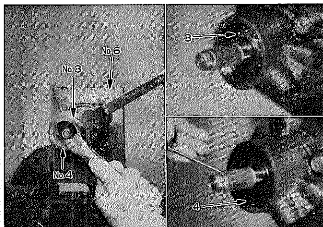
図12-135 ロック ナットおよびアジャスタ プラグ取りはずし H0289 H0288 H0287
