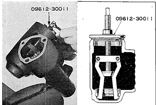
図12-70 ベアリング カップ取りはずし
