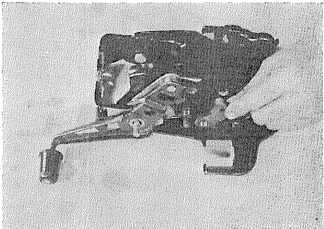
図12-55 チルト ステアリング ポール取り付け
