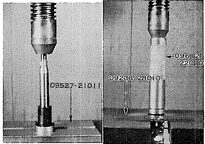
図12-45 ローベアリング交換
