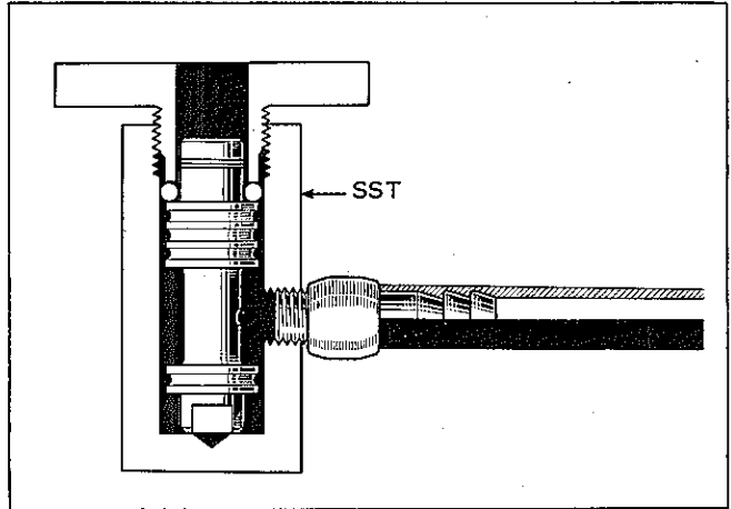
図12-111 油漏れ試験
