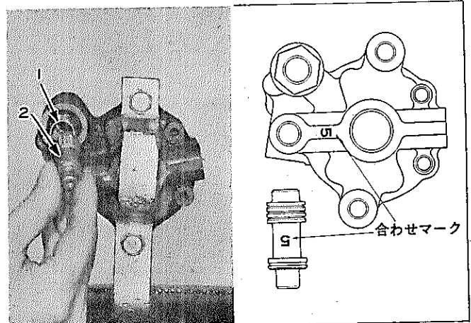
図12-115 コントロールバルブ組み付け
