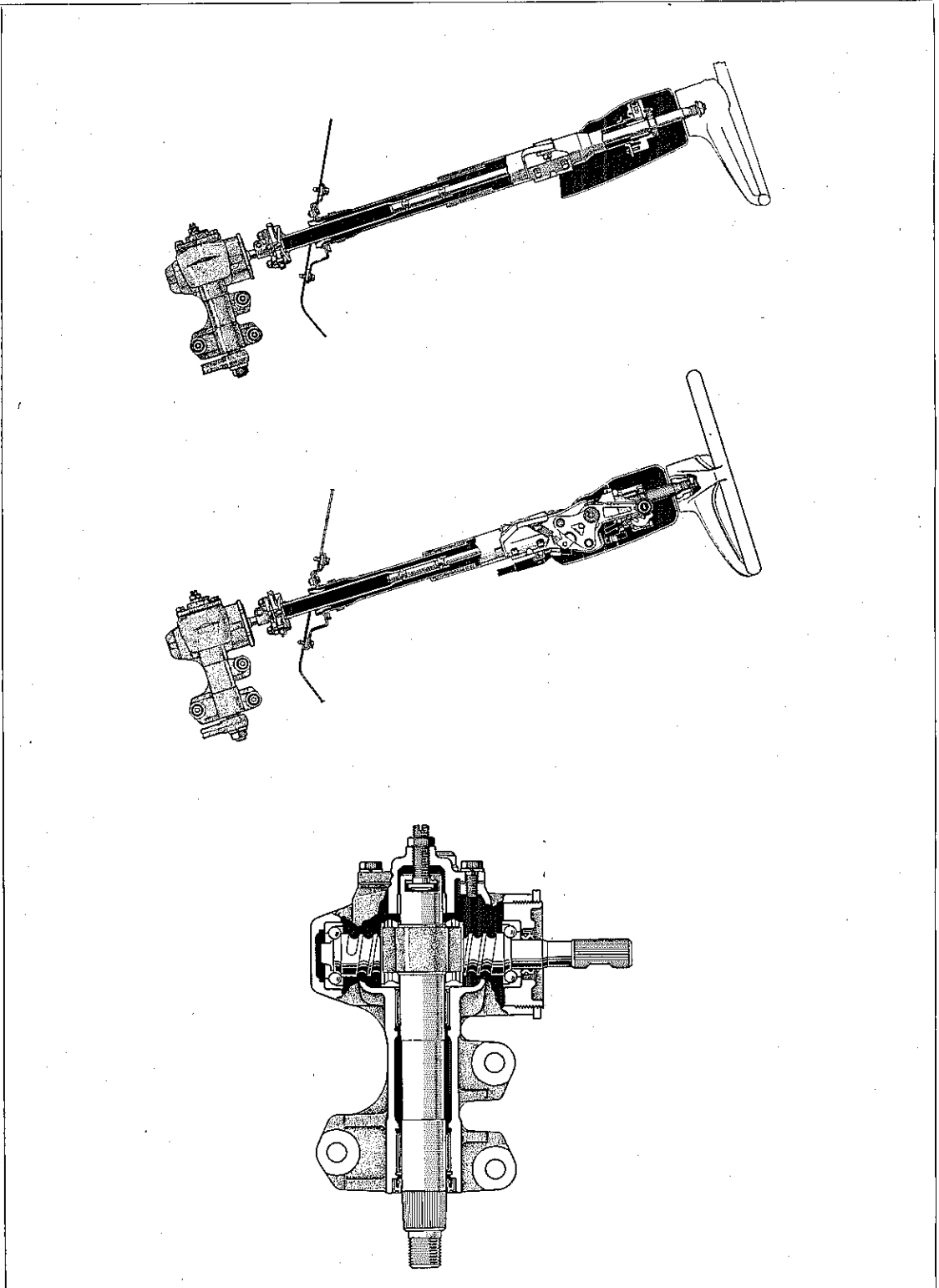
図12-1 断面図
