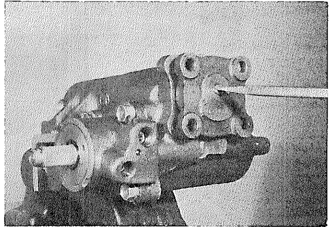
図12-130 エンド カバー取りはずし (その2)
