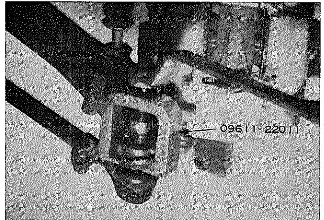
図12-163 タイ ロッド エンド取りはずし
