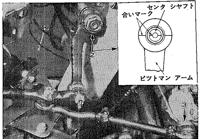
図12-172 組み付け
