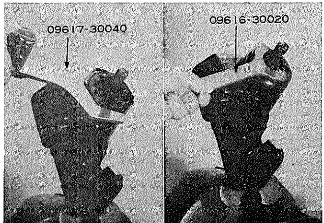
図12-63 ロック ナツトおよび アジャステイング スクリユ取りはずし
