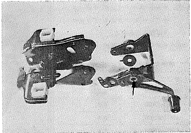
図12-49 チルト ステアリング サポートとブレーク アウエイ ブラケット切り離し
