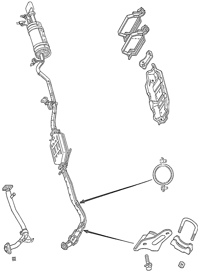
図3-1 排気系統 (4M-EU, M-EUエンジン)
