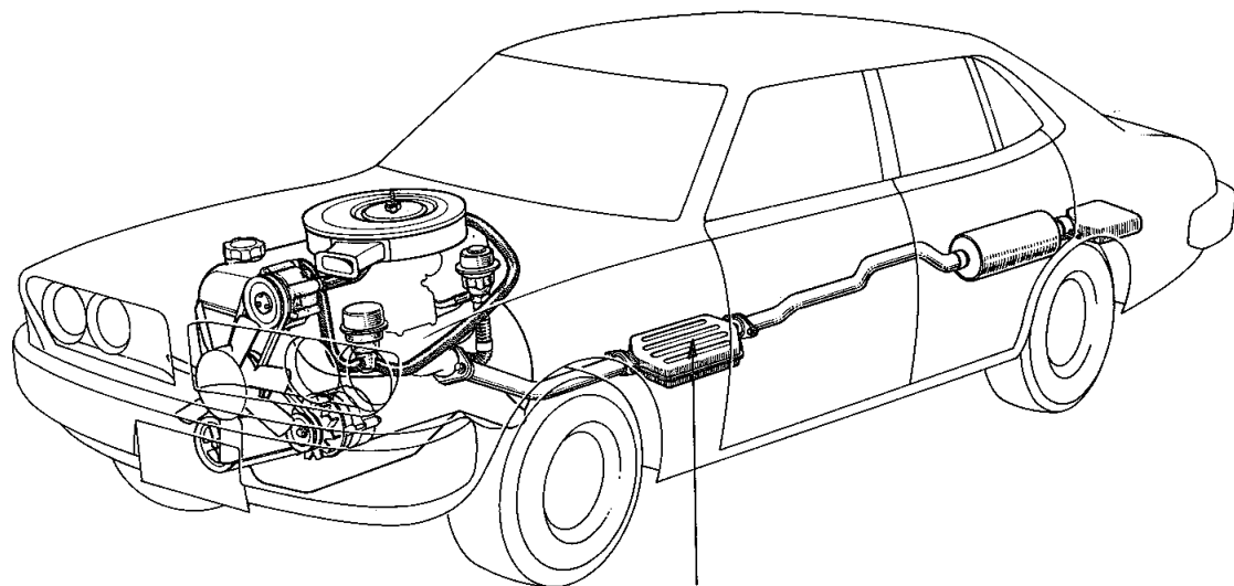
触媒装置
