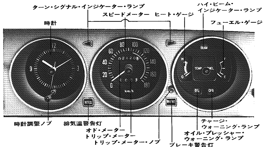
3眼メーター DX, G L, L A車
