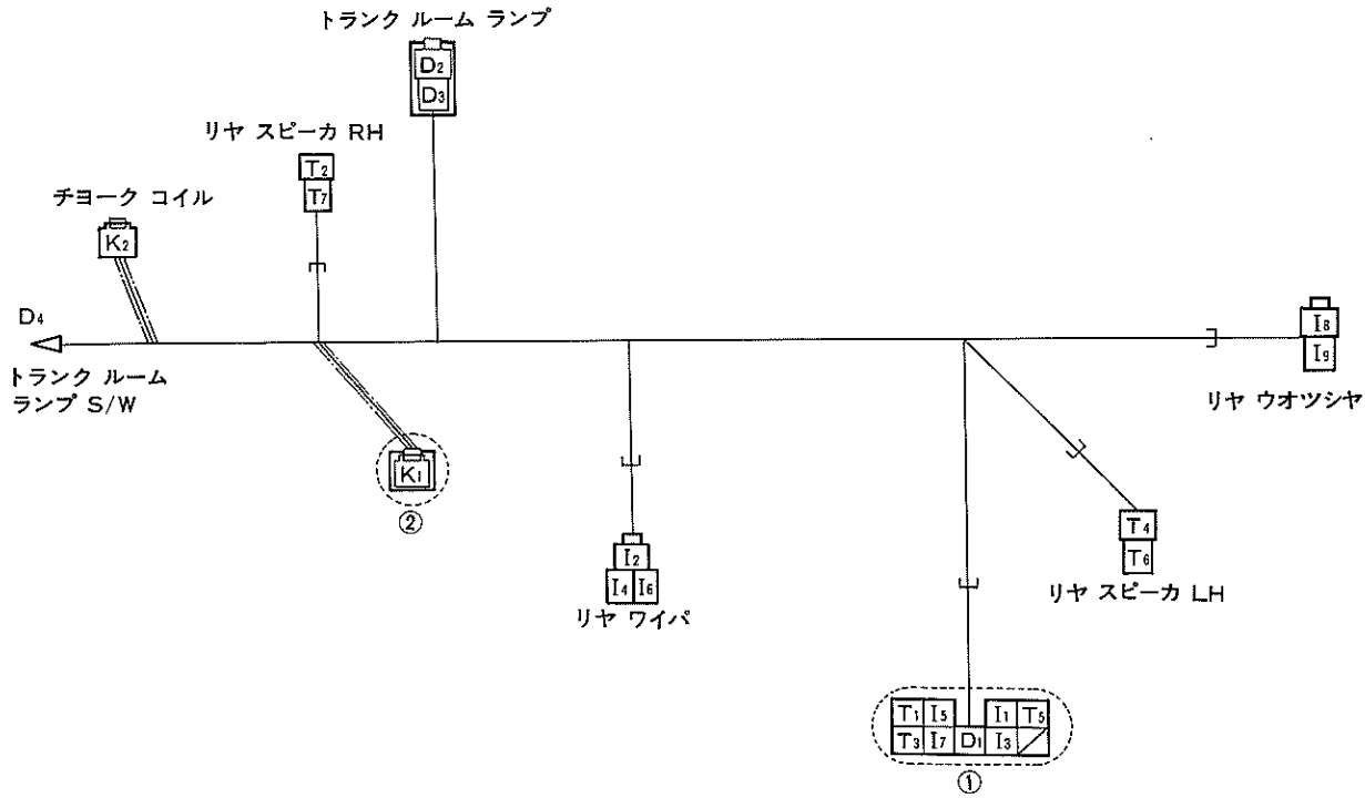
図7-1 ハーネス ASSY, ワイヤリング ツウ リヤ ランプ (セダン-グランデ)
