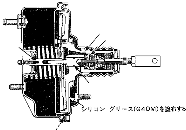
図13-30 グリス塗布個所
