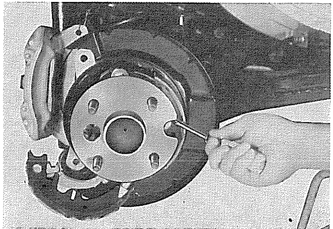
図13-114 ブレーキ シユール取りはずし（その1）
