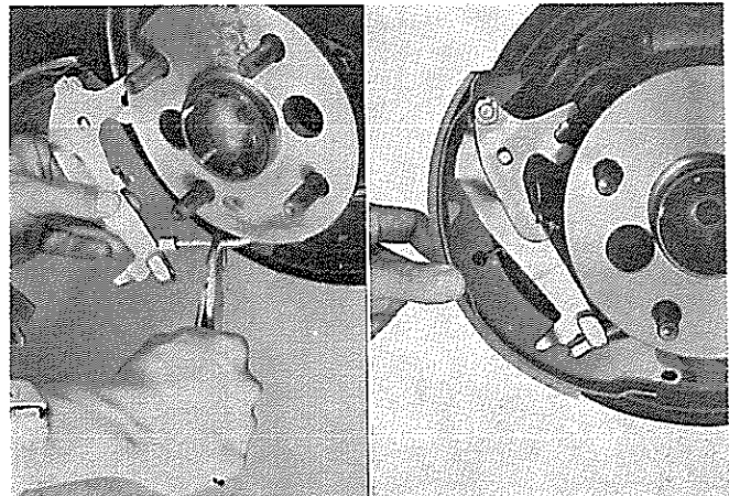
図13-87 ブレーキシュー取り付け(その1)
