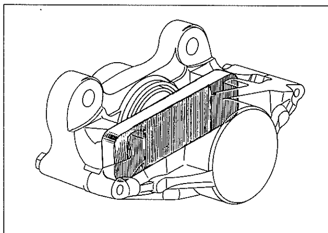
図13-65 ピストン取りはずし
