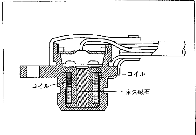
図13-142 断面図
