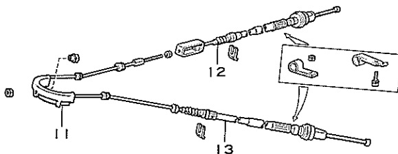
図13-129 構成部品および締め付けトルク
