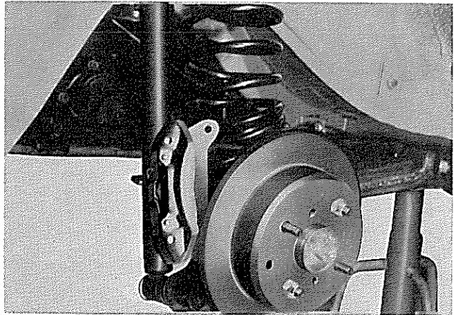
図13-112 キャリパ取りはずし
