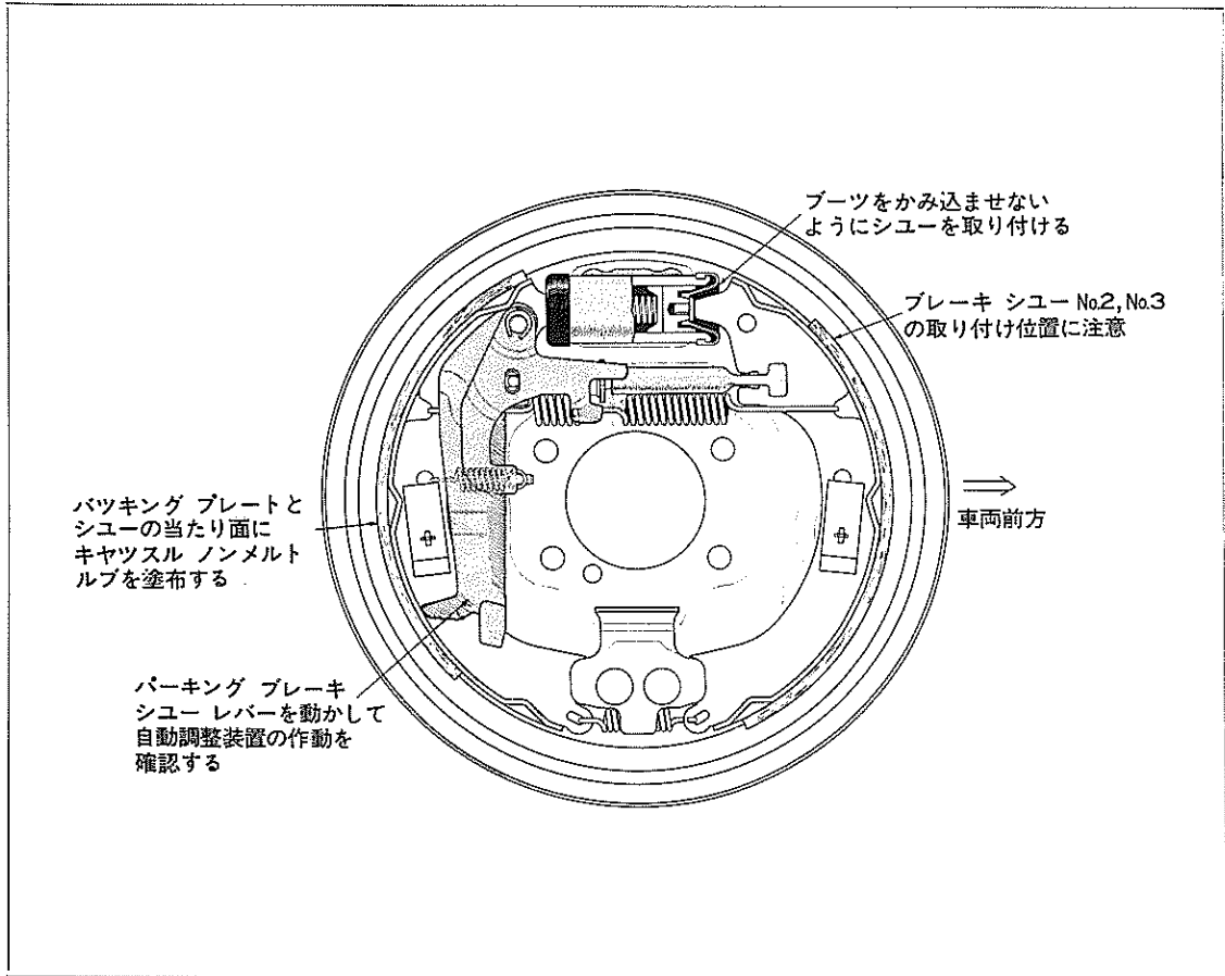
図13-91 リヤ ブレーキ組み付け
