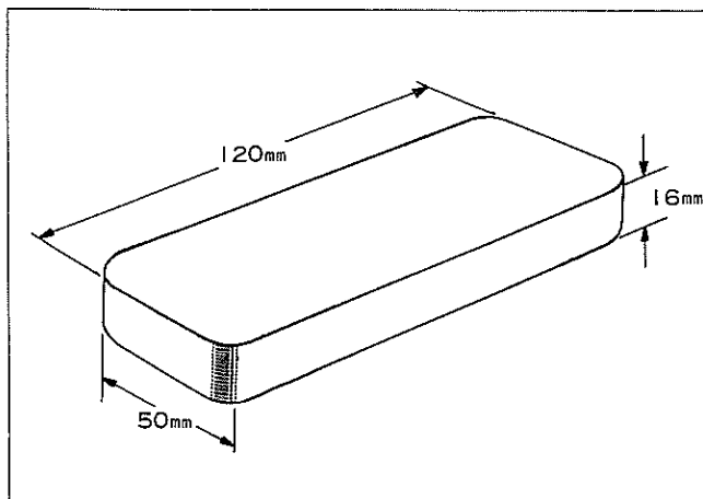
図13-64 当て板
