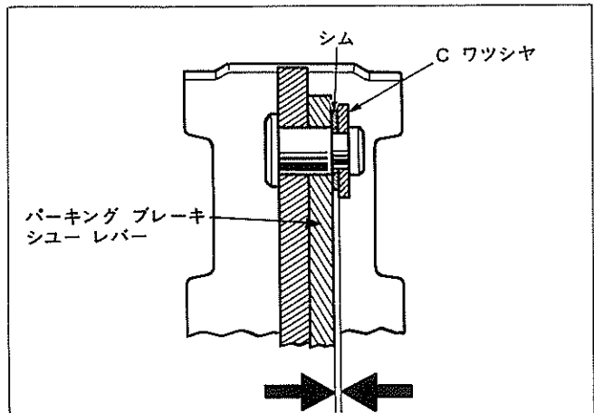
図13-119 パーキング ブレーキ シュー レバー調整 S5816
