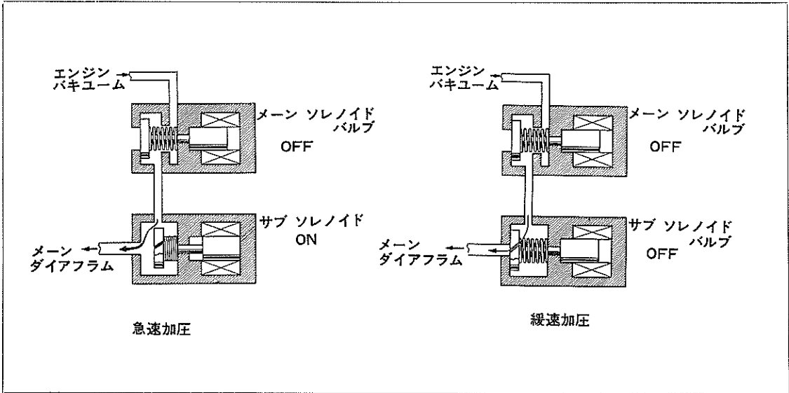
図13-148 メーン ソレノイド、サブ ソレノイドの作動
