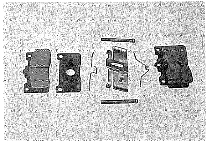
図13-98 点検
