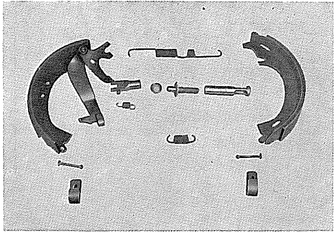
図13-83 点 検
