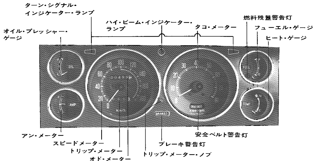
6眼メーター付車……GSL, L, LX, LG
