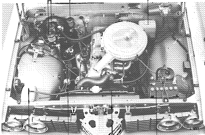
リザーブ・タンク エンジン・オイル・レベル・ゲージ ラジエーター バッテリー
