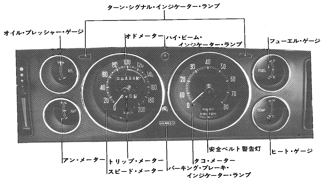
<上の写真はGSS車の計器盤です。>
