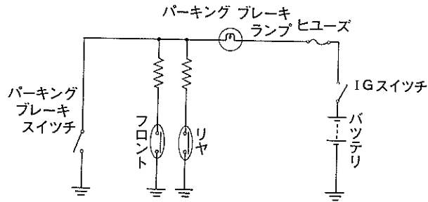
図6-1 回路図
