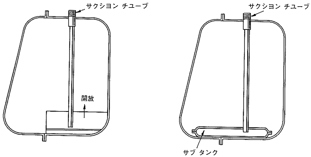
図12-3 フューエル タンク断面
