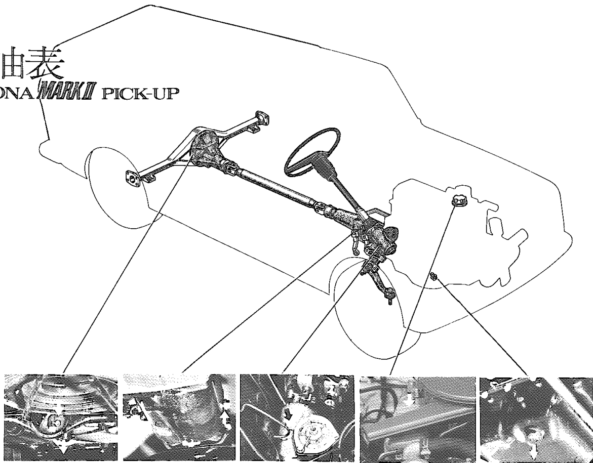
デフアレンシヤル 〈ハイポイド・ギヤ・オイル〉
