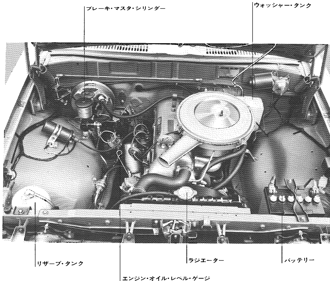
エンジン・オイル・レベル・ゲージ
