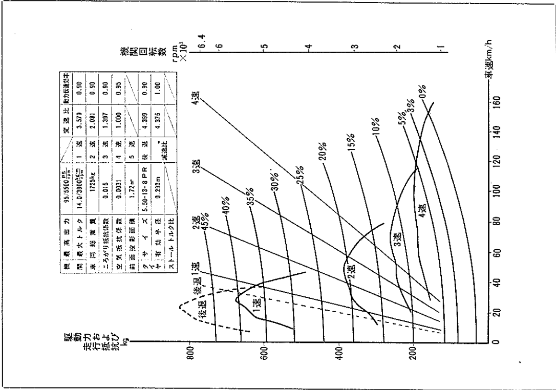
第0-36図 RX16V-KD 型車
