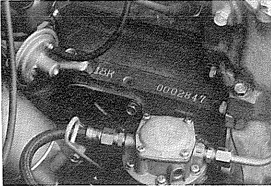
第0-41図 6R, 18R型エンジンNo. 打刻位置 C0053
