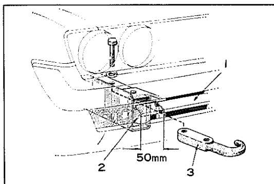
第0-46図 フロントけん引時
